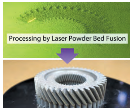
金属粉末にレーザーを照射し造形する金属3Dプリンティング
