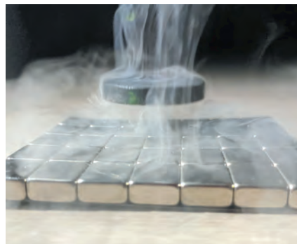
完全反磁性効果により磁気浮上する超伝導体
